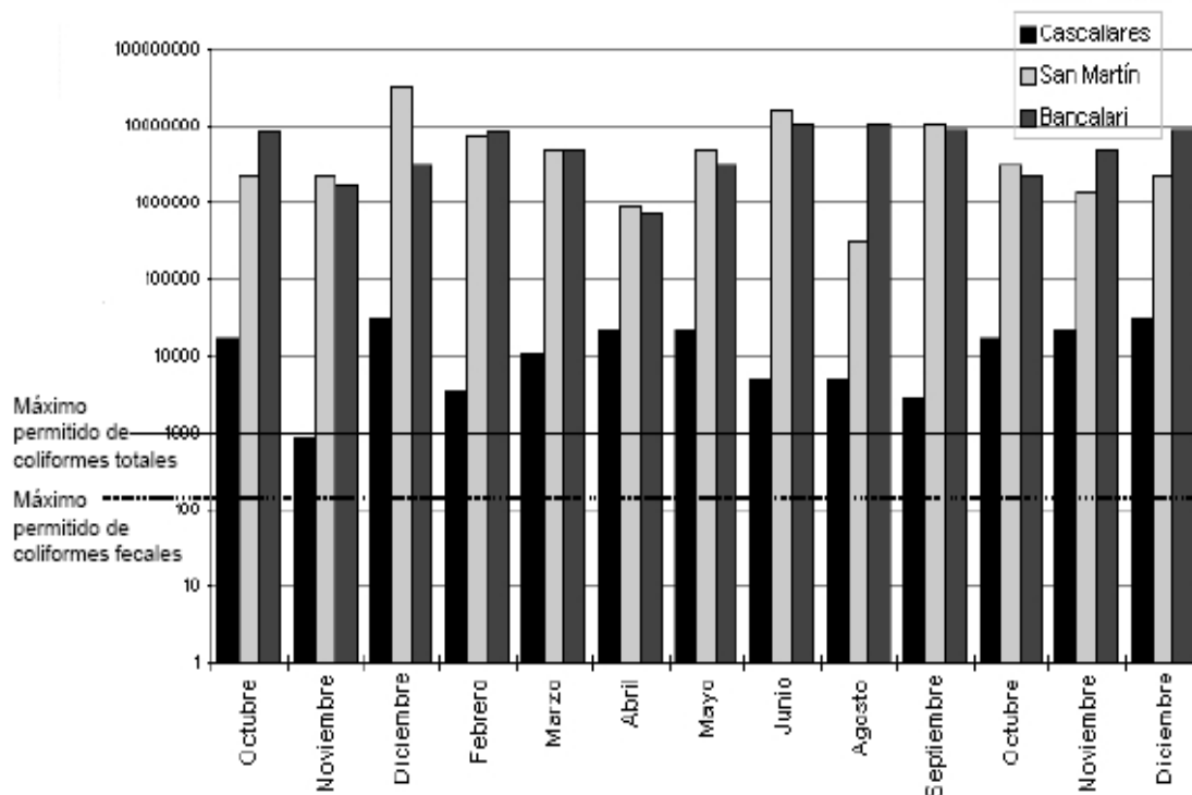
FIGURA 5: BACTERIAS EN MUESTRAS DE AGUA DEL RIO RECONQUISTA. Se presenta la cantidad de bacterias cada 100 ml. Adaptada de Martínez y Salibián 1995 ayb
