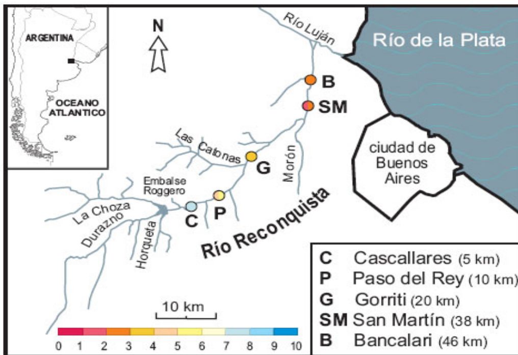
FIGURA 3: ÍNDICE DE CALIDAD DE AGUA por contaminación orgánica (ICA). En los casos en que se detectaron diferencias entre años, la mitad del círculo de la izquierda corresponde al valor del '94 y la de la derecha al del '95.
