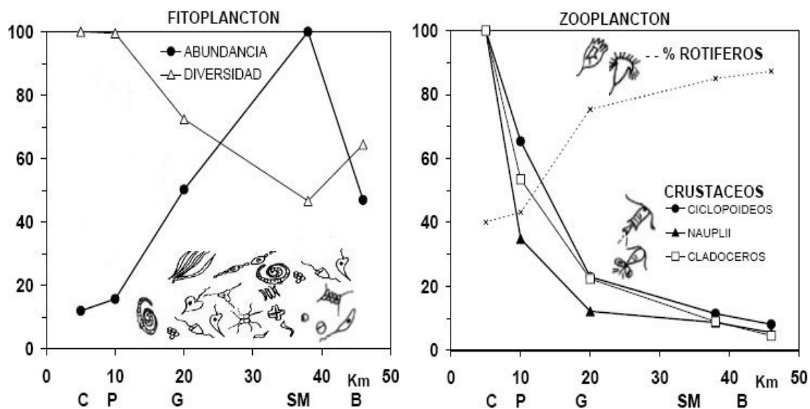
FIGURA 6. VARIACION A LO LARGO DEL RIO DE LA ABUNDANCIA PROMEDIO (1994) DE PLANCTON. Se ubica cada sitio (C: Cascallares, P: Paso del Rey; G: Gorriti; SM: San Martín; B: Bancalari) según su distancia (km) a la naciente del río. a. Valores relativos (porcentajes con respecto al máximo) de densidad y diversidad de algas del fitoplancton; b. Valores relativos (porcentajes con respecto al máximo) de grupos de crustáceos, y proporción de rotíferos en el zooplancton.
