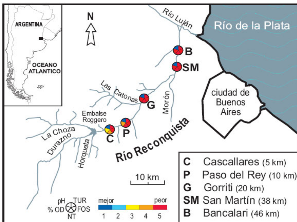
FIGURA 2: Calificación físico-química de las aguas del rio reconquista según los criterios sepa
