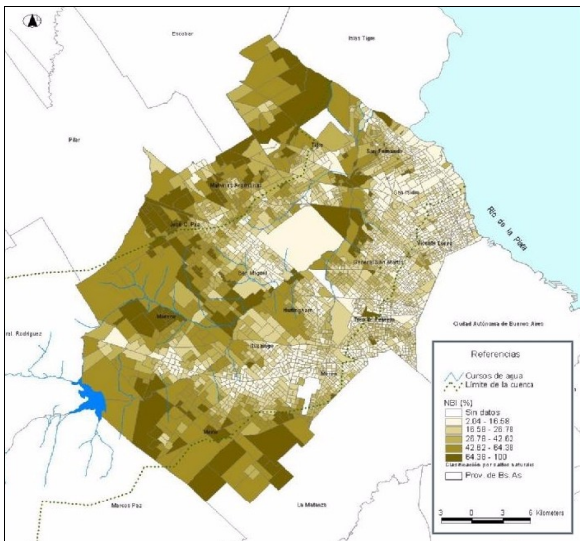
FIGURA 2: Porcentaje de población con NBI en los partidos de la cuenca, por radio censal. Tomado de Sadañowski 2003
