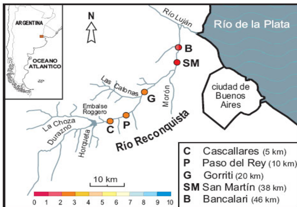
FIGURA 4: ÍNDICE DE CALIDAD DE AGUA POR CONTAMINACIÓN INDUSTRIAL (ICAPI). En los casos en que se detectaron diferencias entre años, la mitad del círculo de la izquierda corresponde al valor del '94 y la de la derecha al del '95.
